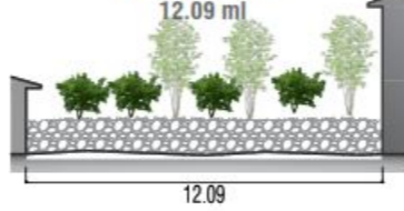
CORTE 52-52 PASAJE S/N 06 VIA SIN AFIRMAR 12.09 ml
